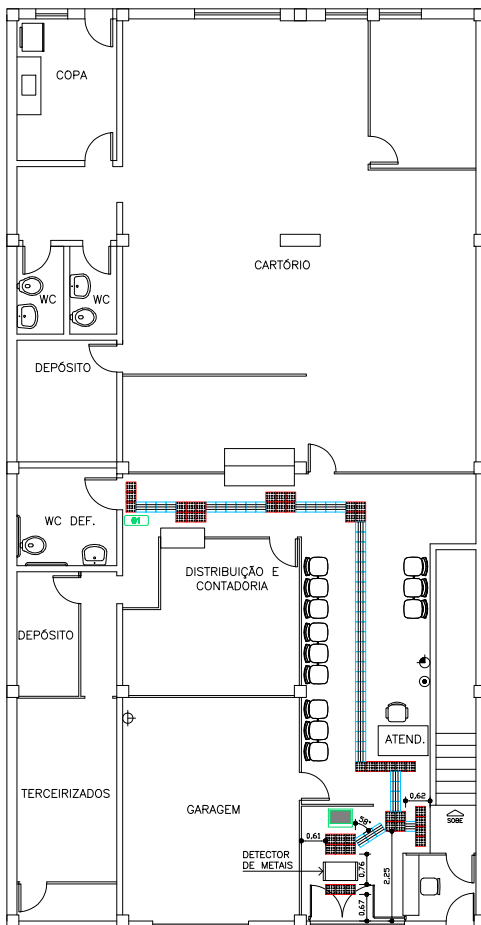
PL. BAIXA PAV. TÉRREO - SINALIZAÇÃO TÁTIL ENC. 1/18
