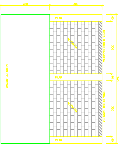
VISTA FRONTAL DO MURO – SEÇÃO 2
