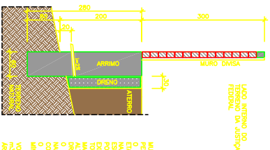
CORTE – SEÇÃO 2
