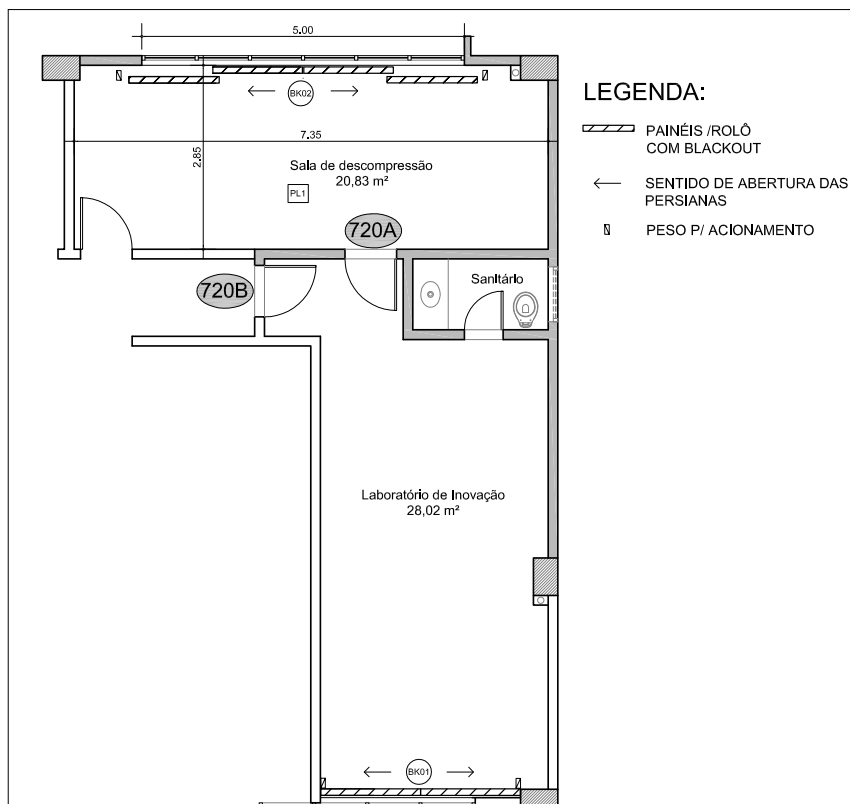
PLANTA BAIXA - LABORATÓRIO DE INOVAÇÃO
