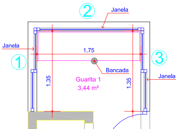
GUARITA 1 - PL. BAIXA ESCALA 1/25
